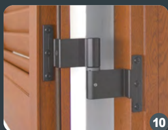
→ Cerniera su telaio con superamento della spalletta (anta aperta)
