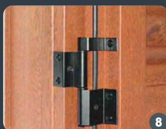
→ Cerniera su telaio a due ali con antisfilamento (anta aperta)
