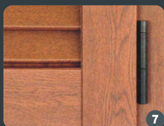
→ Cerniera su telaio a due ali con antisfilamento (anta chiusa)
