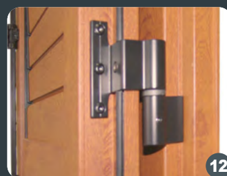
→ Cerniera su anta primaria per pacchetto esterno (anta aperta)
